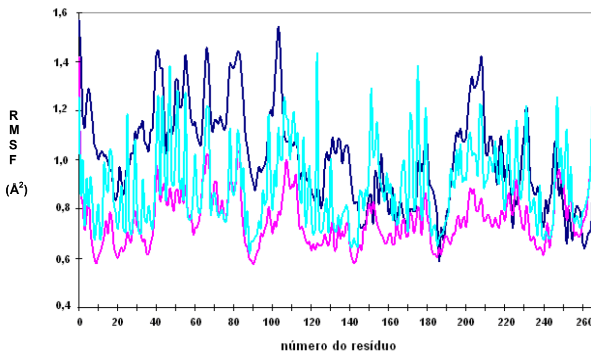
Figura 3.8 - Gráfico do RMSF da cadeia principal da InHA a 25 °C (magenta) e a 37 °C (ciano) em comparação com o RMSF da estrutura inicial (azul escuro). Os valores estão mais elevados na estrutura cristalográfica do que nas simulações.
