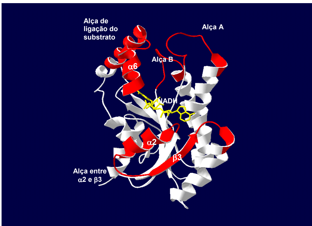
Figura 3.9 Representação das regiões de maior mobilidade da estrutura cristalina da InhA (cód. 1ENY). Os resíduos que compreendem a Alça A são de 100 a 114; a Alça B, de 150 a 161; a alça de ligação do substrato, de 197 a 220. Os resíduos 41 a 69 constituem a hélice \alpha_2 , a fita \beta_3 e a alça que está compreendida entre as duas estruturas.
