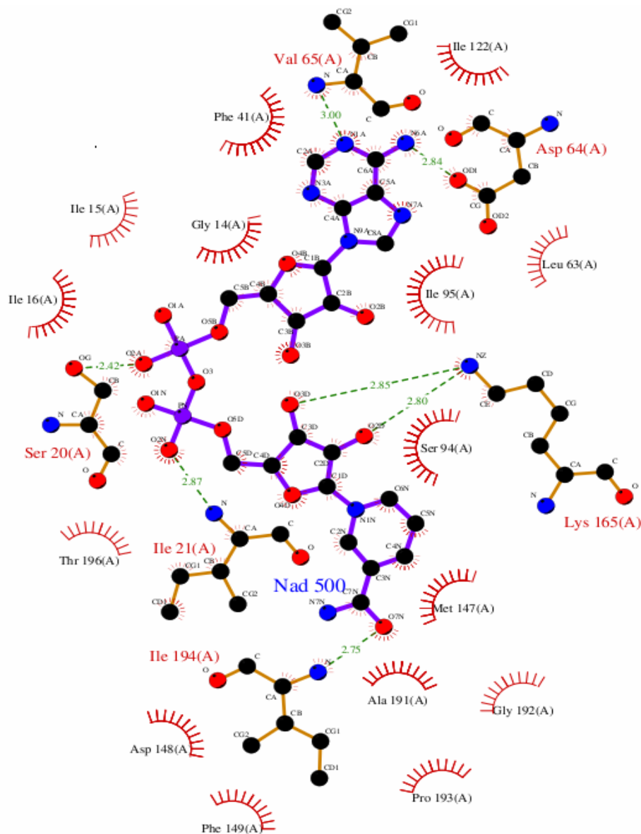
Figura 3.17 – Estrutura cristalina da InhA (cód. pdb: 1ENY) mostrando a interação entre o NADH e os resíduos da proteína. Figura obtida através do programa LIGPLOT (Wallace et al., 1995).
