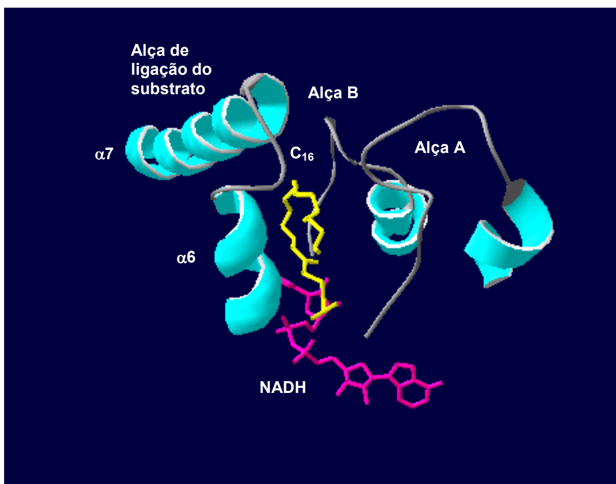
Figura 1.5 Representação do tipo ribbons das alças A e B e de alça de ligação do substrato da InhA (hélices \alpha 6 e \alpha 7 ). Entre as alças visualizam-se o análogo do substrato C_{16} e, na região inferior, a coenzima NADH (código PDB: 1BVR - subunidade C).
