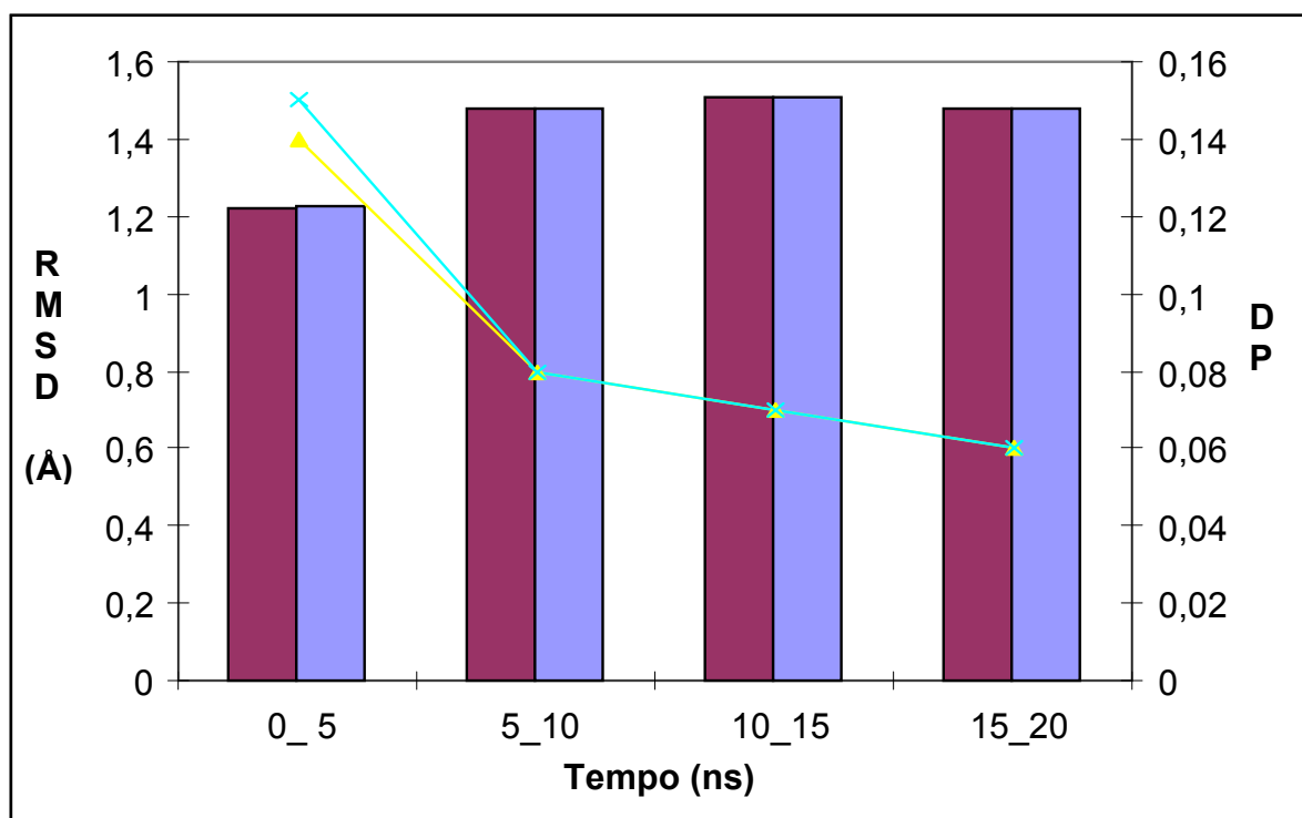
Figura 3.4 Gráfico das médias (colunas) e desvios padrões (DP - linhas) do RMSD das simulações por DM em ambas as temperaturas. O segmento de 15 a 20 ns mostra o menor DP do RMSD em relação aos outros intervalos de tempo.
