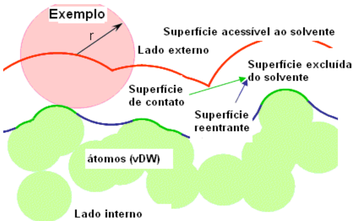
Figura 3.5 Modelos de superfície molecular. Em vermelho, temos uma linha que delimita a ASAS. A linha verde corresponde aos contatos de van der Waals: em conjunto com a linha azul, representa a superfície molecular (SM). Figura extraída e adaptada de Voss et al. (2006).
