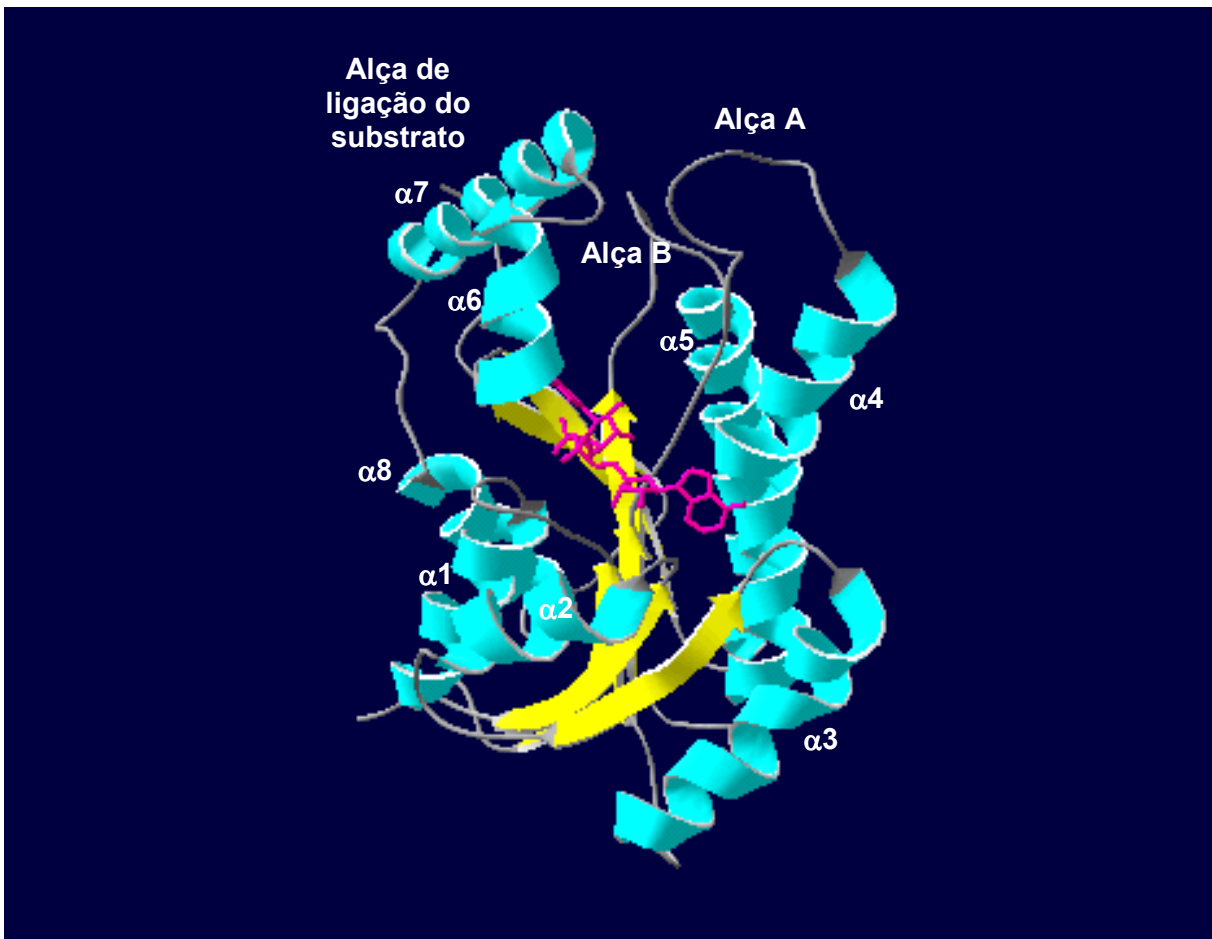
Figura 1.3 Representação do tipo ribbons da cadeia principal da estrutura terciária da enzima InhA de Mycobacterium tuberculosis . As oito hélices \alpha (em ciano), flanqueiam a folha \beta (em amarelo) constituída de sete fitas. A coenzima NADH (magenta), encontra-se em uma conformação estendida acima do núcleo formado pela folha \beta . Encontram-se destacadas as alças A (resíduos 100 a 114), B (resíduos 150 a 161) e de ligação ao substrato (resíduos 197 a 204 da hélice \alpha 6; resíduos 209 a 220 da hélice \alpha 7) (código PDB: 1ENY – Dessen et al., 1995).
