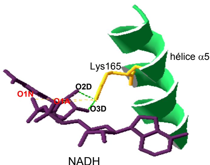
Figura 3.19 – Visualização da coenzima NADH, resíduo Lys165 e parte da hélice \alpha 5 na estrutura cristalina 1ENY. As linhas verdes tracejadas representam as ligações de H que ocorrem entre o resíduo Lys165 e os átomos O2D e O3D da porção nicotinamida do NADH. Estas ligações também são observadas nas estruturas resultantes das simulações por DM aos 25 °C. Aos 37 °C, por outro lado, a Lys165 passa a ligar-se ao NADH através de ligações de H com os átomos O1N e O1A da porção pirofosfato (linhas tracejadas em amarelo). Optou-se por utilizar uma imagem da estrutura cristalina da InhA (pdb 1ENY) ao invés de estruturas resultantes das simulações por DM por conseguir uma imagem mais nítida desta região e dos resíduos envolvidos na interação.
