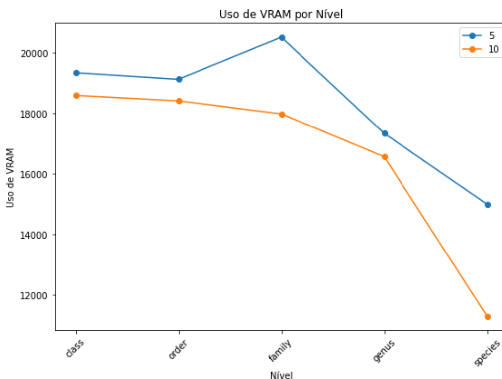
Figura 6.3: Uso de VRAM de cada limite mínimo, para cada nível.
