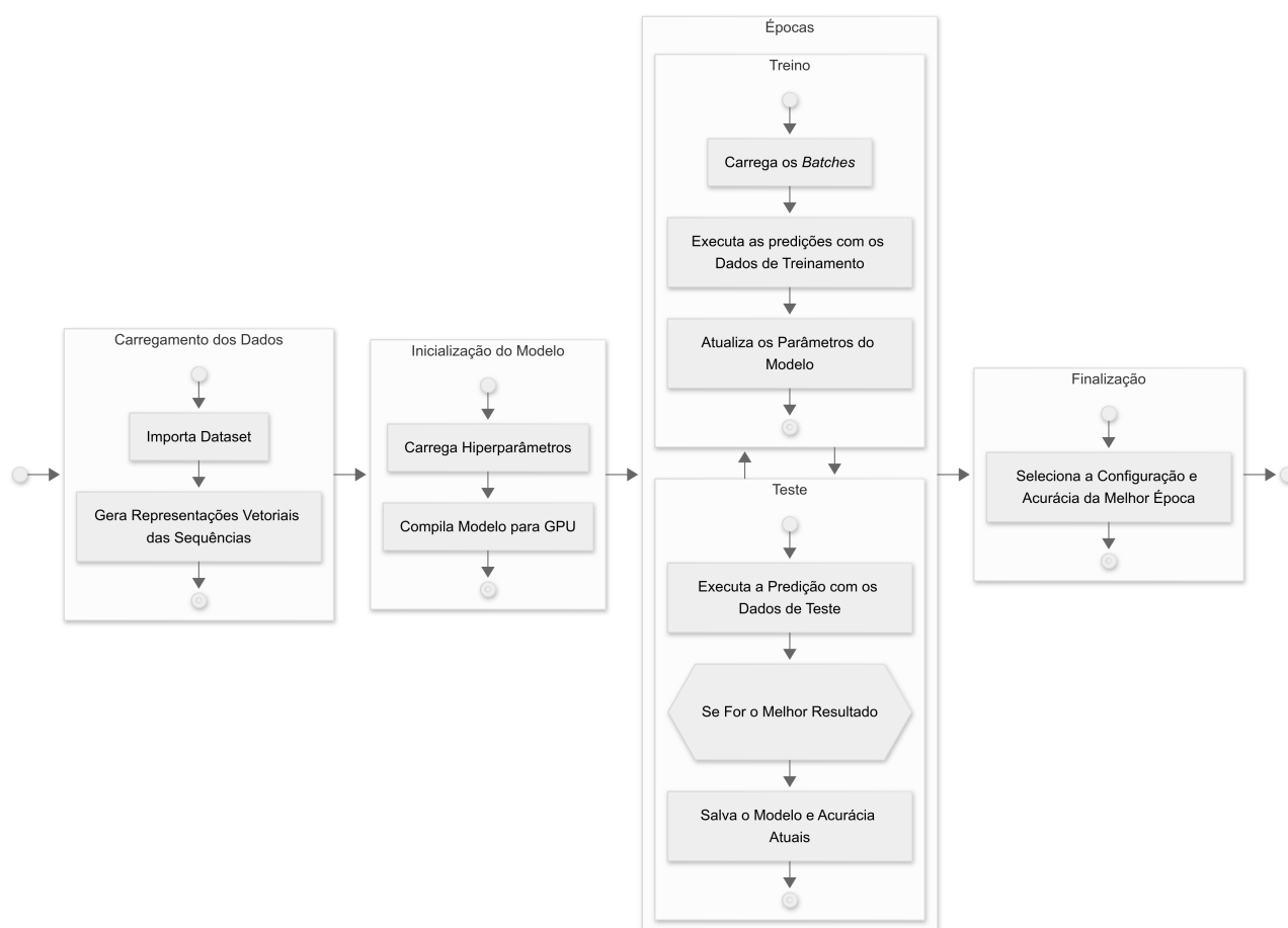
Figura 6.2: Diagrama da execução dos experimentos com a solução desenvolvida.
