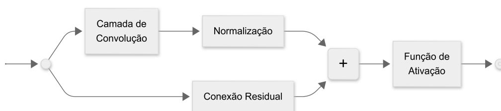
Figura 5.2: Diagrama do bloco de camada convolucional.
