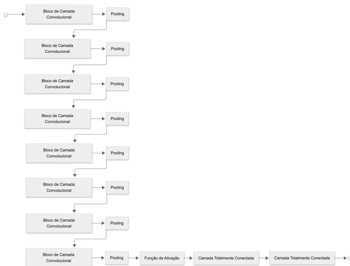
Figura 5.1: Diagrama da arquitetura do modelo.
