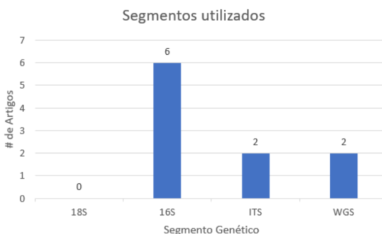
Figura F.2: Gráfico da contagem de artigos que utilizam cada um dos segmentos genéticos.
