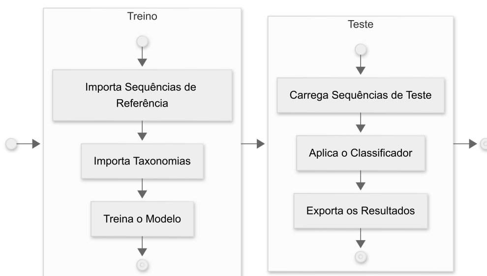
Figura 6.1: Diagrama da execução do plug-in q2-feature-classifier.
